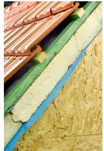
Bauteile wie Dächer, Aussenwände oder Zwischendecken müssen in der Regel F90 sein. Sie bestehen aus mehreren Schichten und Materialien mit unterschiedlicher Brennbarkeit. Quelle: Alterfalter/ Fotolia
